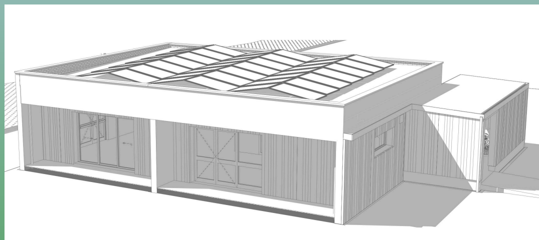
Bâtiment commercial Saint-Jean Trolimon 36 m 2 - 7 kWc - 21 panneaux
