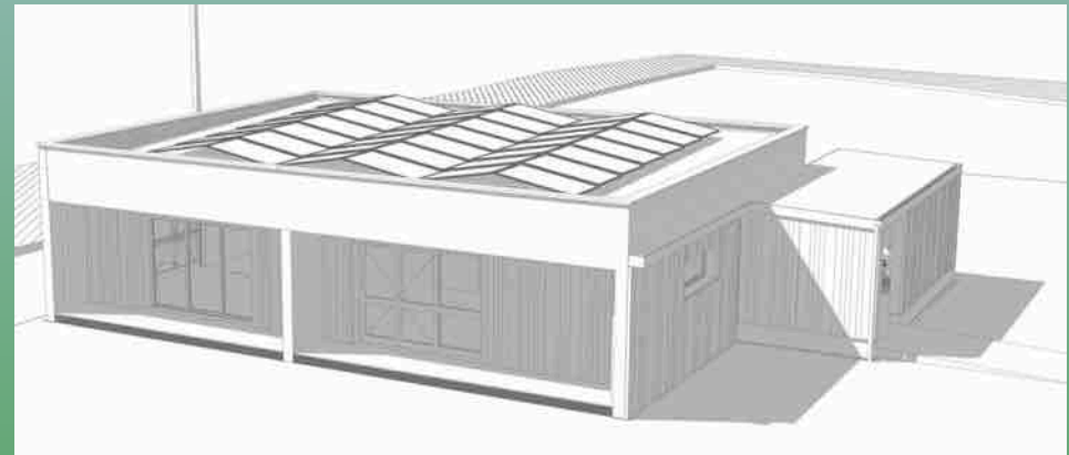
Espace Jeunes de Combrit Puissance 17 kWc - 42 panneaux Début des travaux Février 2023
